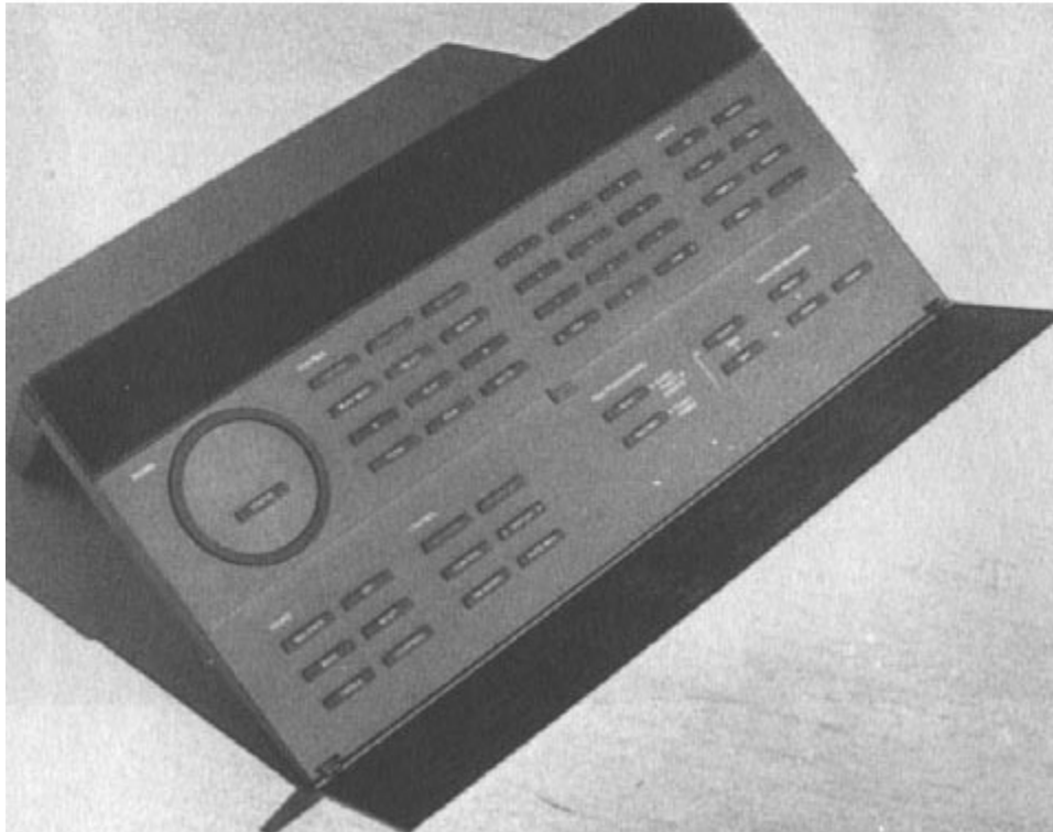
Рис. 6.9. Преодоление сложности через организацию. Дистанционный пульт управления (вверху) к комплекту аудиоаппаратуры Bang&Olufsen (на самой аппаратуре нет никаких элементов управления) предоставляет широкие возможности в
