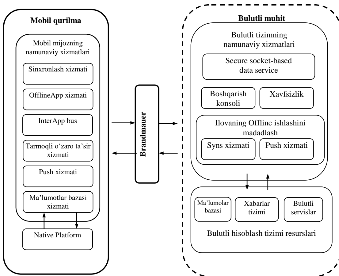
10.1-rasm. OpenMobster platforma arxitekturasi
