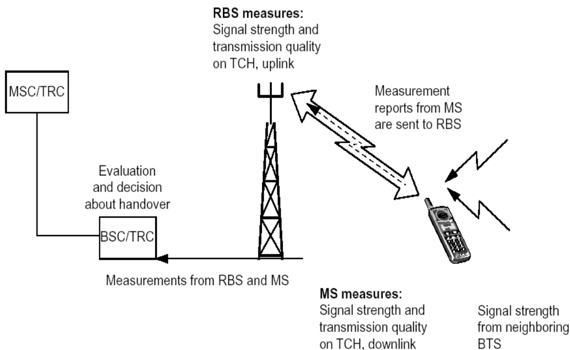
2.21- rasm. BSCga uzatiladigan o‘lchashlar natijalari
