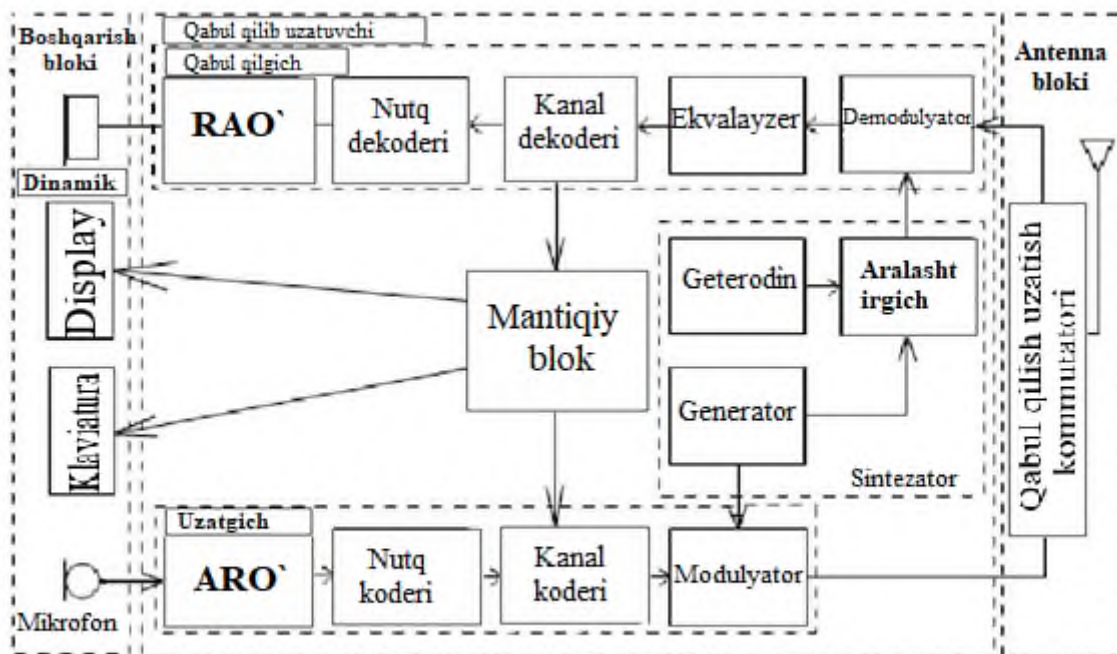
1.2- rasm. Mobil stansiya qabul qilgich-uzatkichining soddalashtirilgan blok-sxemasi
