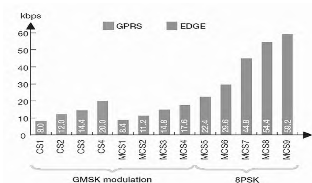
1.6- rasm. GPRS va EDGE texnologiyalaridagi turli kodlash sxemalari
