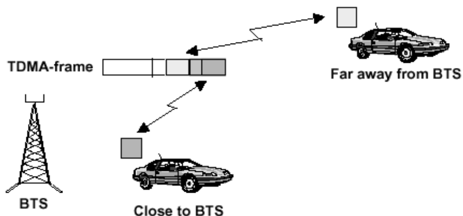
4.15- rasm. Vaqt bo'yicha kechikish
