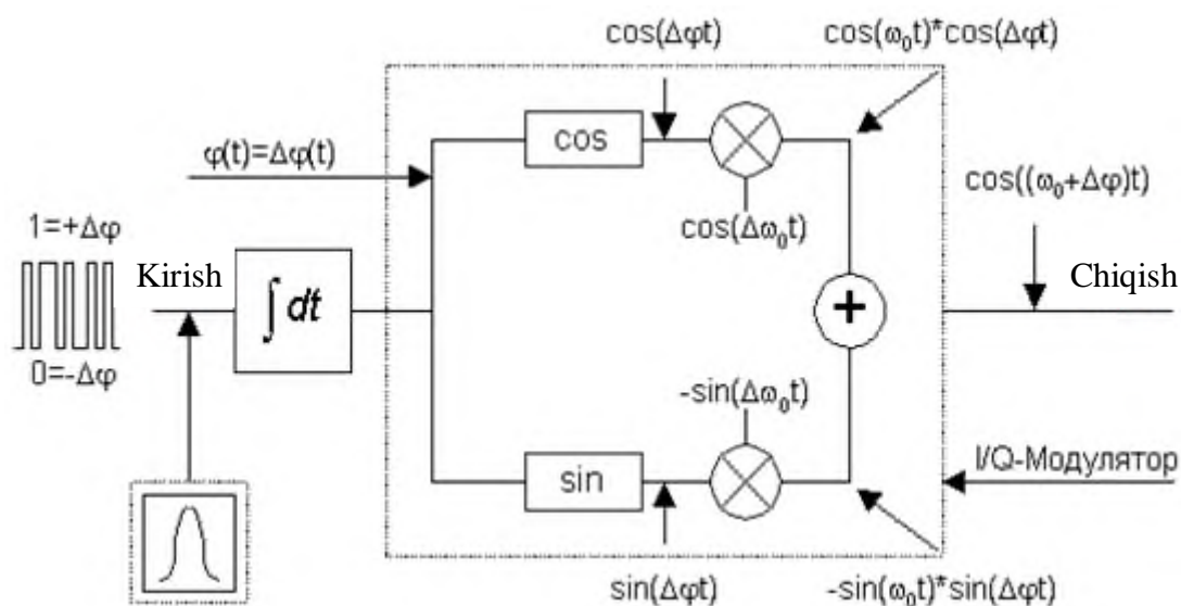
4.11- rasm. GMSK-signalni shakllantirish tamoyili
