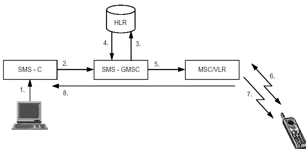
2.27- rasm. Qisqa xabarlarni mobil qabul qilishi
