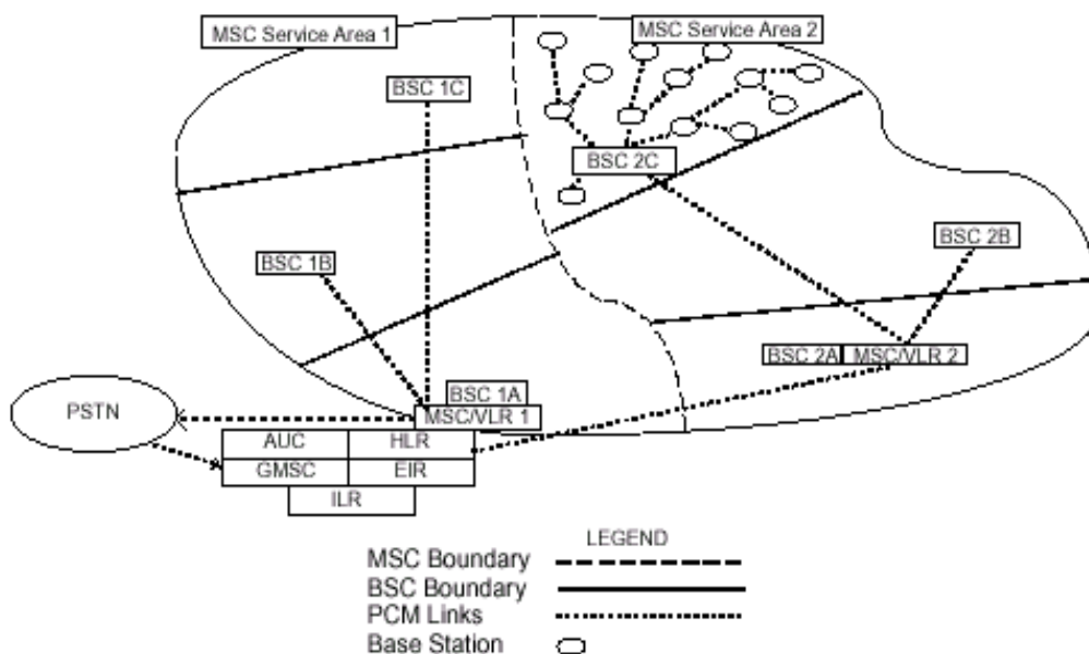
1.11- rasm. Tarmoq tugunlarining joylashishi va ularning apparatlar ta'minoti darajasidagi o'zaro ta'sirlashishi
