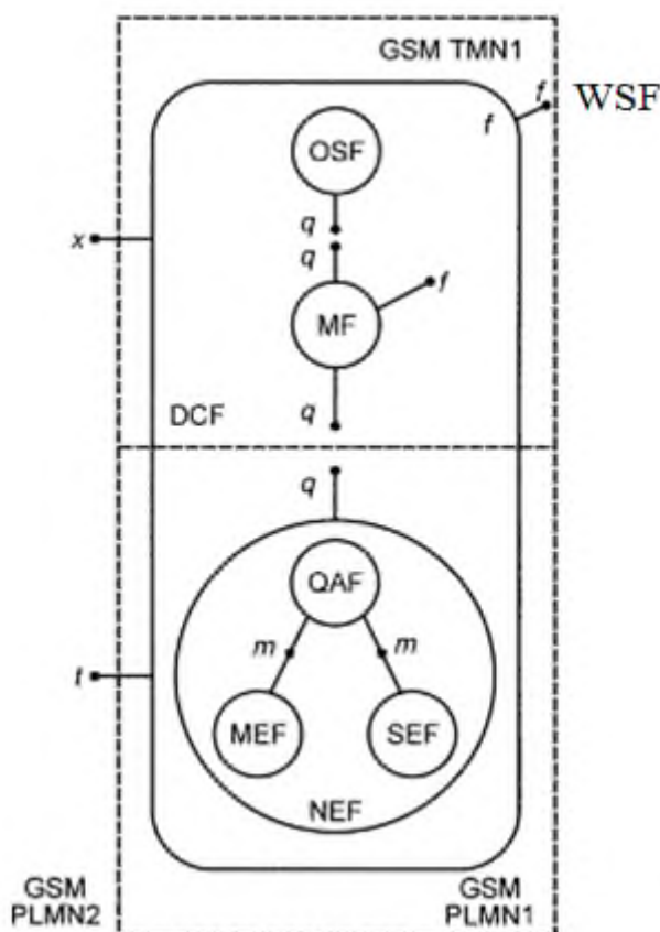
5.1- rasm. GSM tizimida aloqa jarayonlarini boshqarish sxemasi
