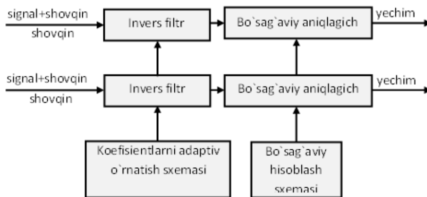
4.9- rasm. VADning tuzilish sxemasi
