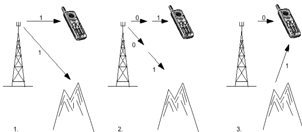
4.14- rasm. Vaqt dispersiyasi
