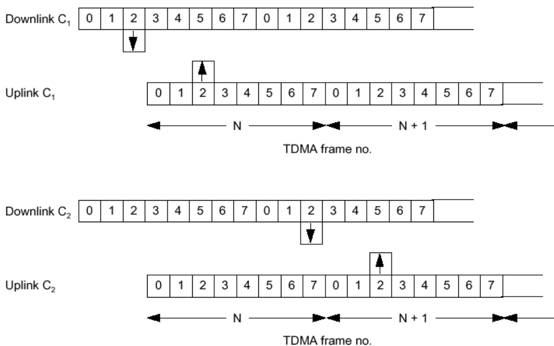
4.22- rasm. Chastota bo'yicha sakrashlar
