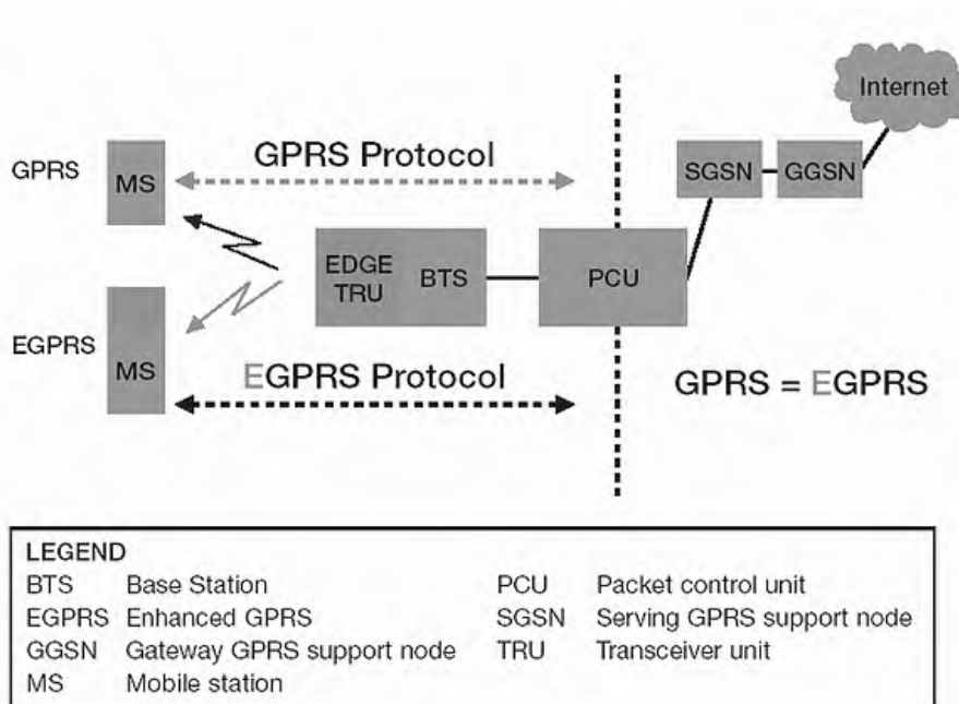
1.1- rasm. EDGE va GPRS texnologiyalari orasidagi farq
